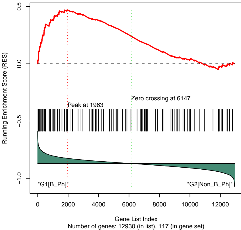
Gene Set 1605 : B_PhvsNon_B_Ph_Hypo
